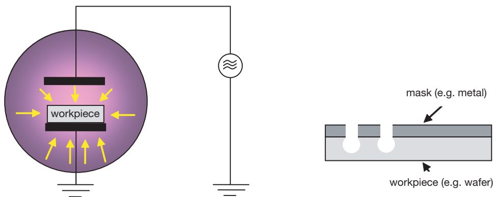
fig. 149: PE operation
